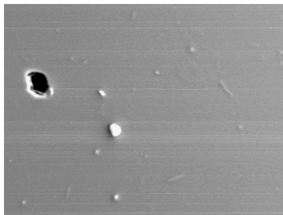
Figura 5. Presencia de “droplets” en la superficie de una película delgada obtenida por PLD.
