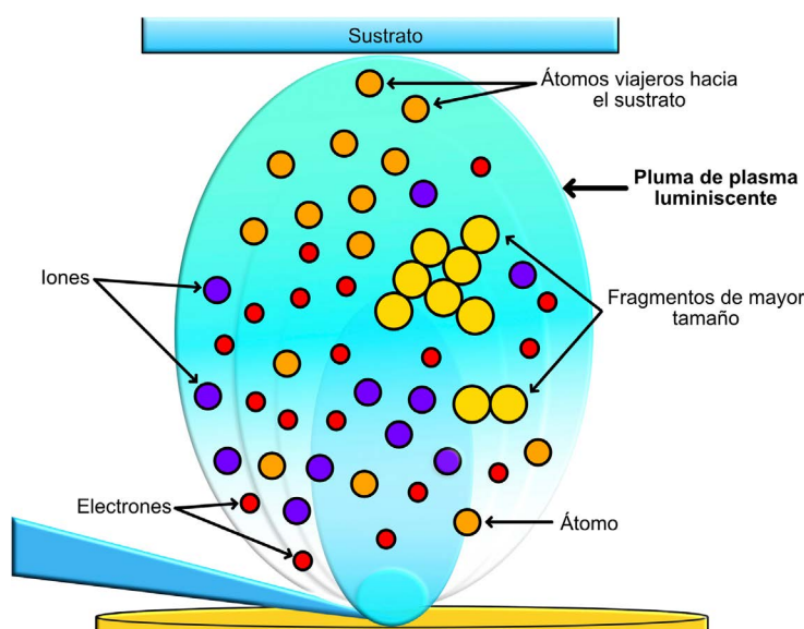
Figura 3. Imagen representativa del plasma formado.
