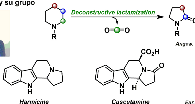
Figura 4. Edición molecular en alcaloides piperidínicos usando nuestra lactamización deconstructiva.
