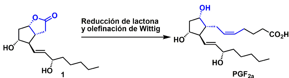
Figura 1. Síntesis de la PGF 2α de Corey como ejemplo de refuncionalización.
