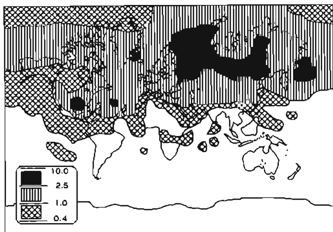
Áreas afectadas por las nubes del invierno nuclear, a 10 días (fig 2a) y a 20 días (fig. 2b) después del conflicto. Las unidades se refieren a profundidad óptica. Las profundidades 2.5
