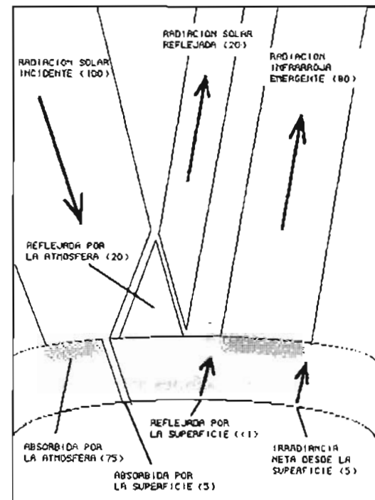
Relaciones de energía incidente y reflejada para el caso de una atmósfera normal (izquierda) y para el caso de una densa nube de polvo y humo (derecha). (R.P. Turco y col, 1983).
