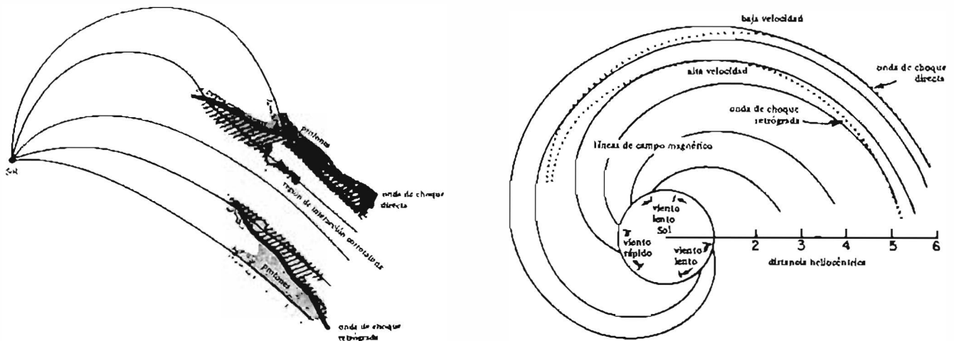
Figura 9. a) Esquema de una región de interacción coronatoria (RIC): las regiones oscuras alrededor de las ondas de choque representan la distribución espacial de protones energéticos (de acuerdo con E. J. Smith). b) RIC vista desde el marco de referencia que corrotta con el Sol (de acuerdo con L.A. Fisk).
