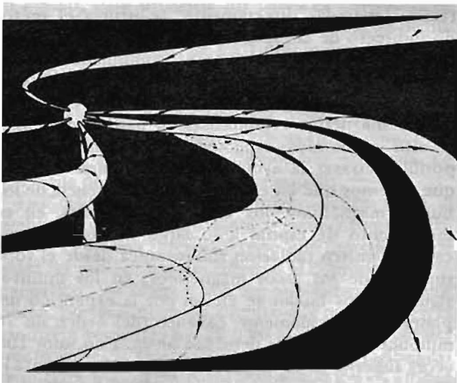
Figura 21. Esquemización de los "tubos" de campo magnético (tubos de Arquímedes) en que se concentran las líneas de campo magnético interplanetario.
